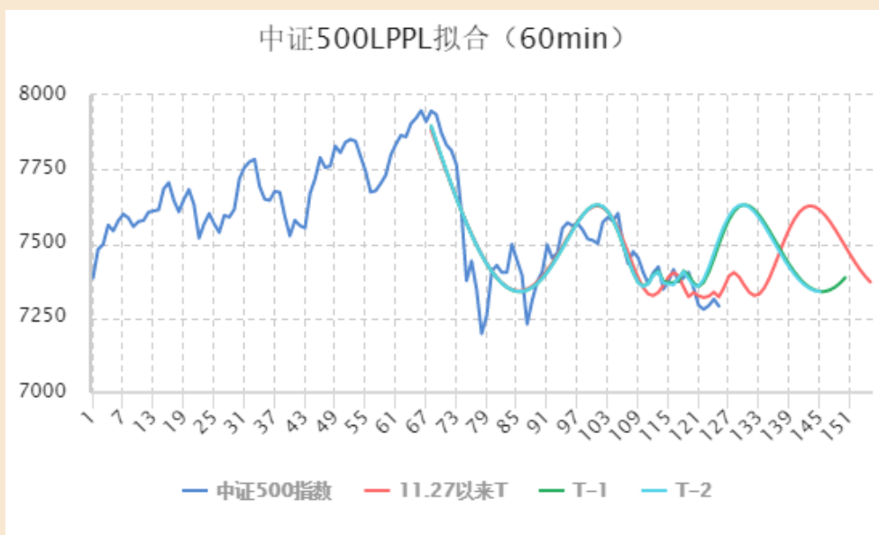
图一 中证500指数实际走势与拟合效果
