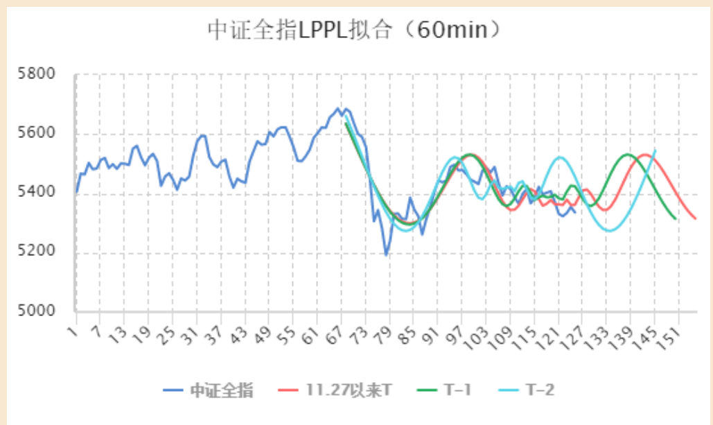
图四 中证全指实际走势与拟合效果
