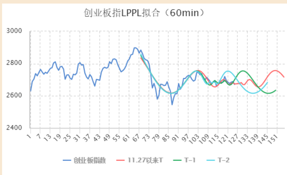
图二 创业板指数实际走势与拟合效果
