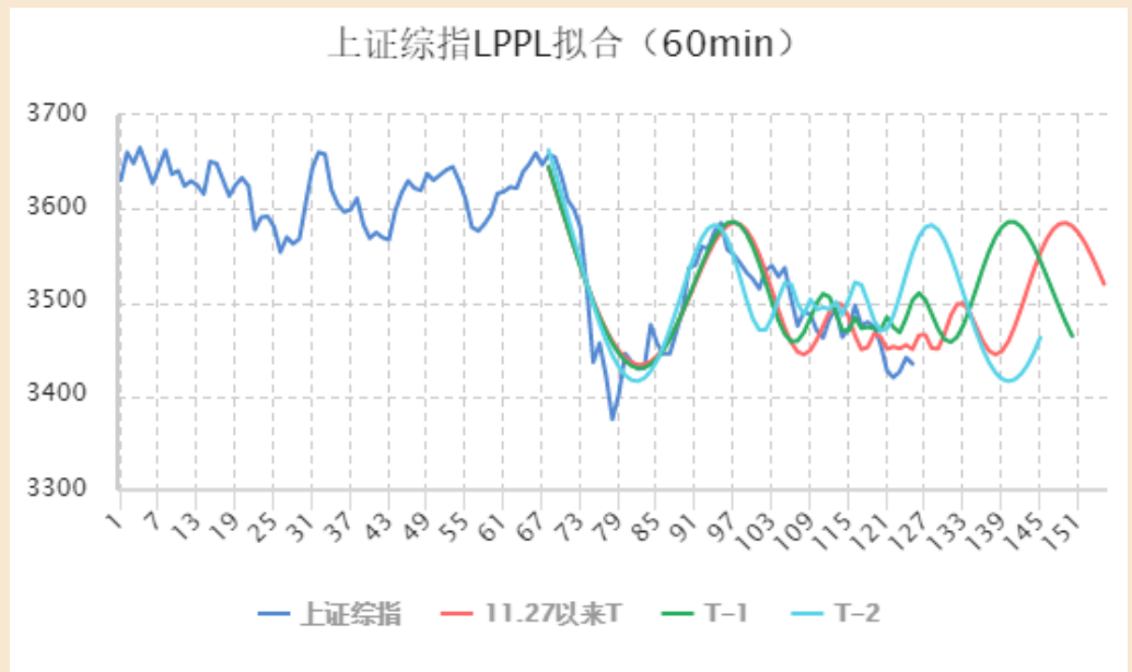
图三 上证综指实际走势与拟合效果
