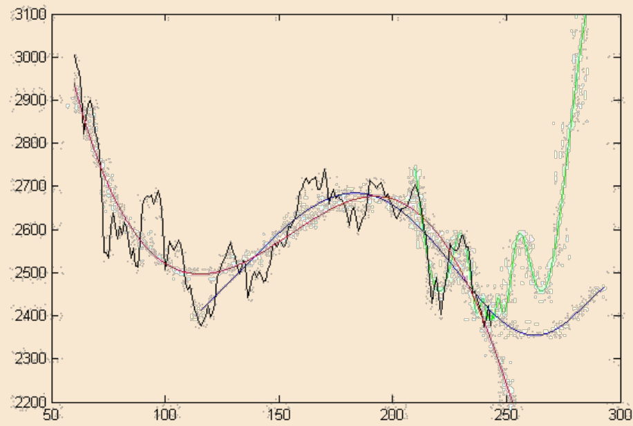
图2 创业板指数30分钟线实际走势与拟合效果图
