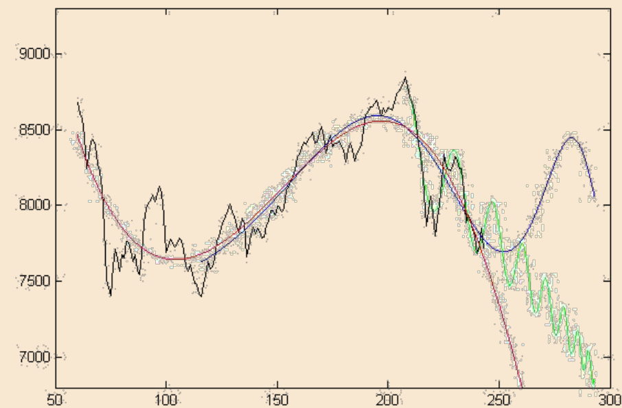
图3 中证500指数30分钟线实际走势与拟合效果图
