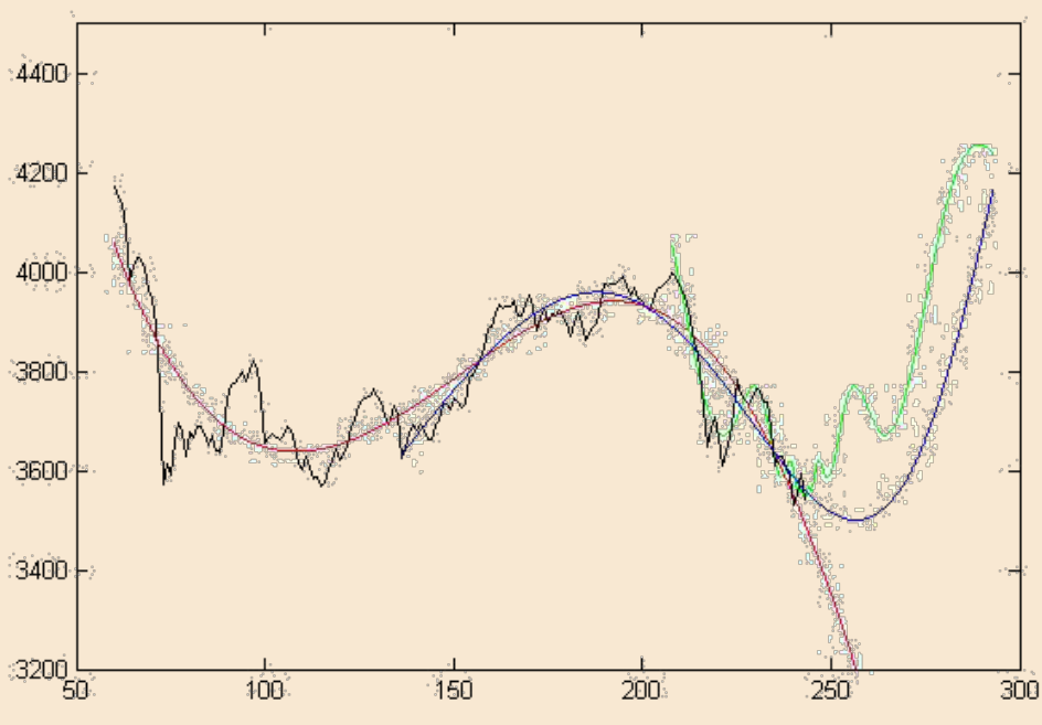
图1 上证指数30分钟线实际走势与拟合效果图
